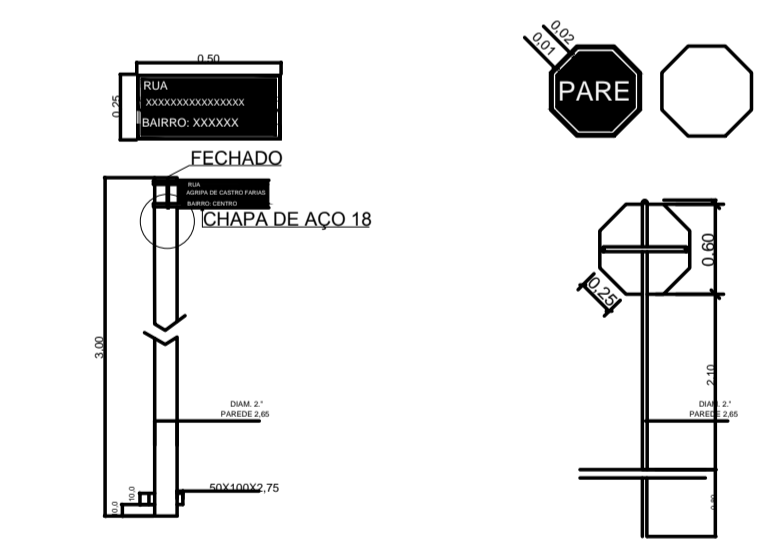
DETALHE DE PLACAS DE REGULAMENTAÇÃO
