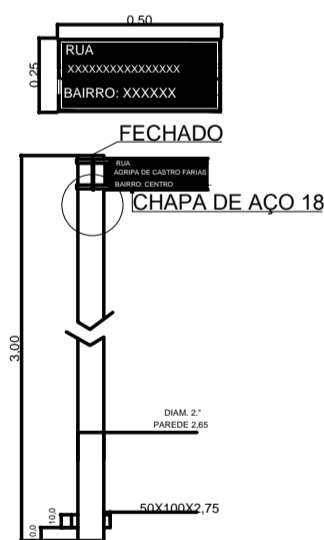
DETALHE DE PLACAS DE REGULAMENTAÇÃO
