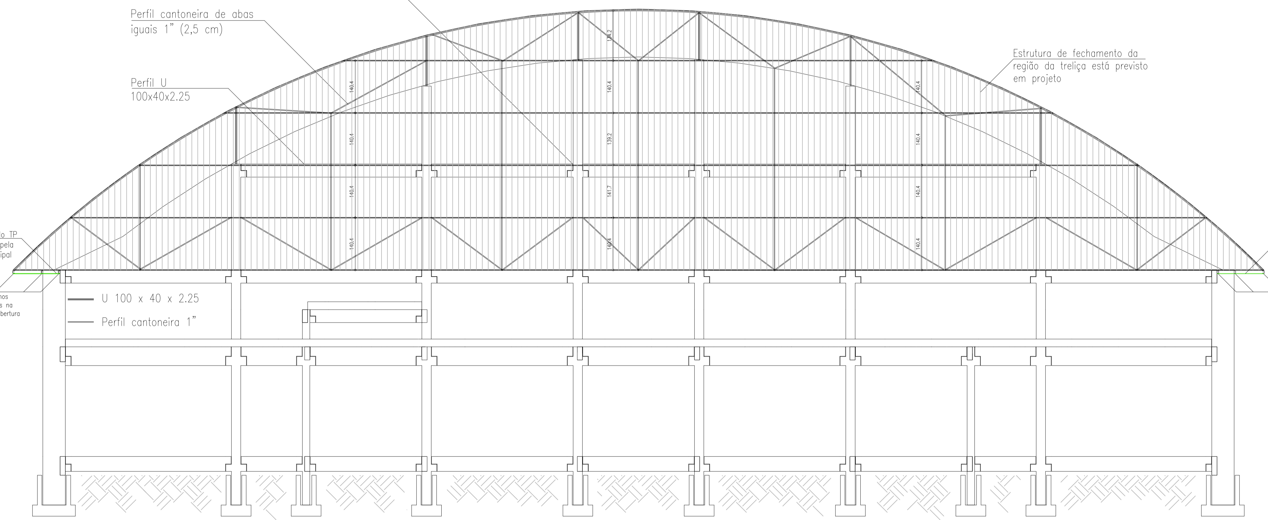
DETALHE GERAL: FECHAMENTO DOS OITÕES E BEIRAIS Escala: 1:50
