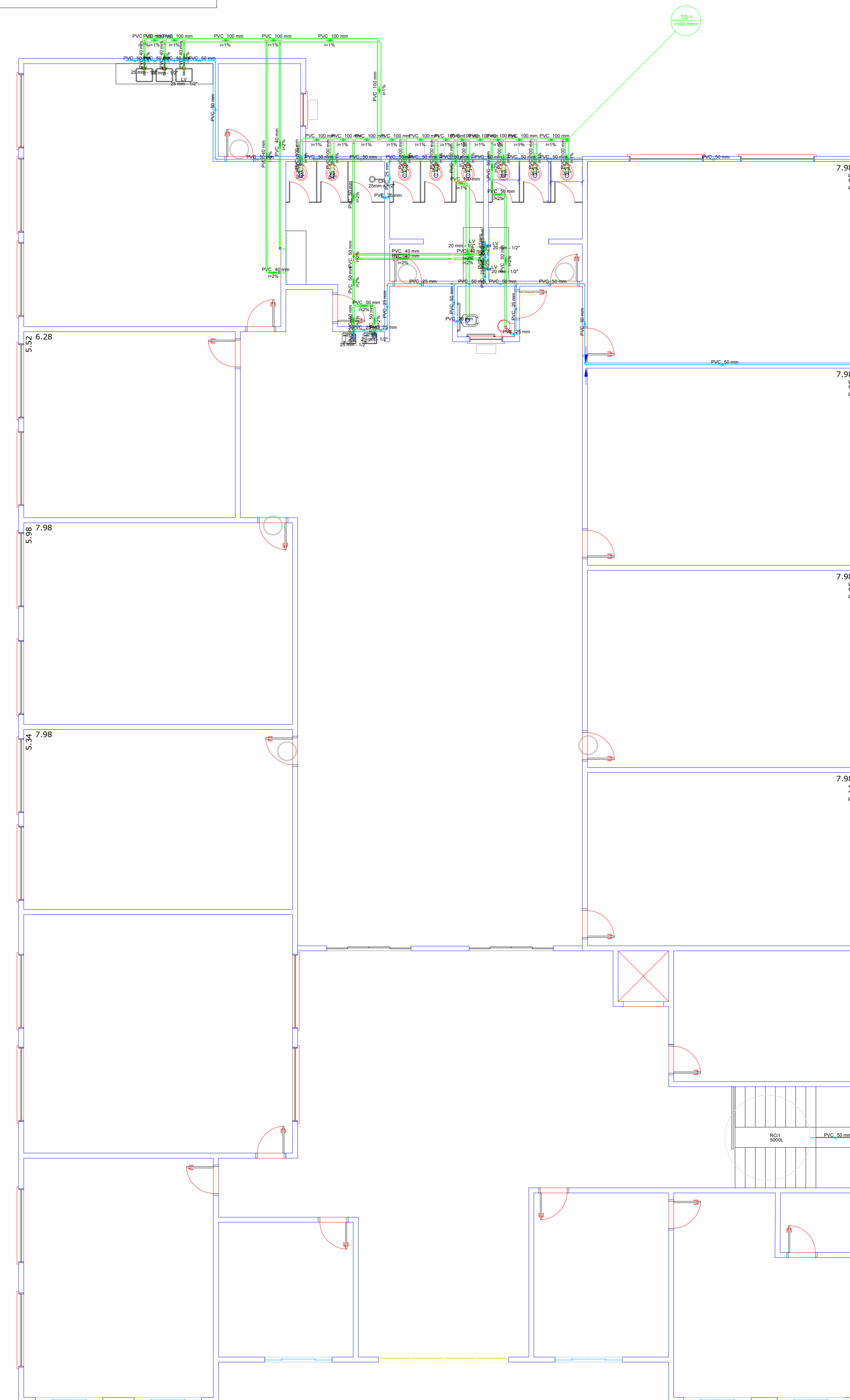
Esquema hidrossanitário (1º Pavimento) ESCALA 1/75
