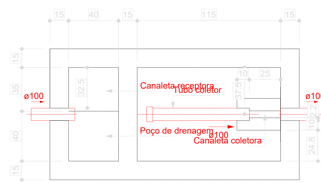
Filtro anaeróbio Planta baixa - ESC. 1:25
