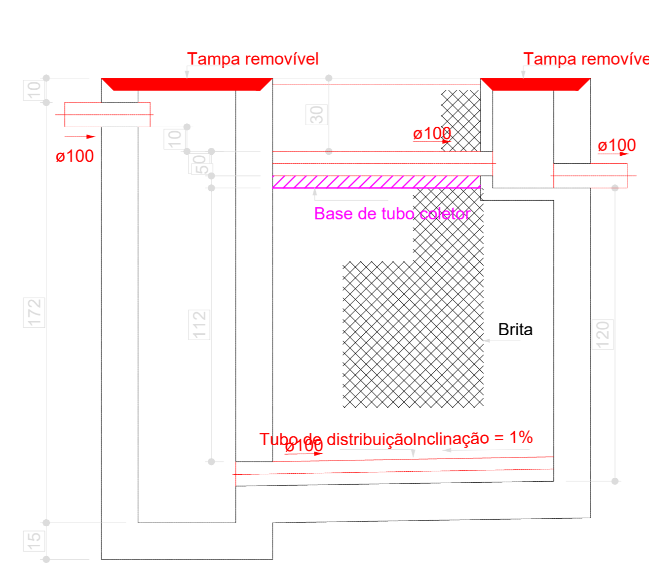
Filtro anaeróbio Corte 1 - ESC. 1:25
