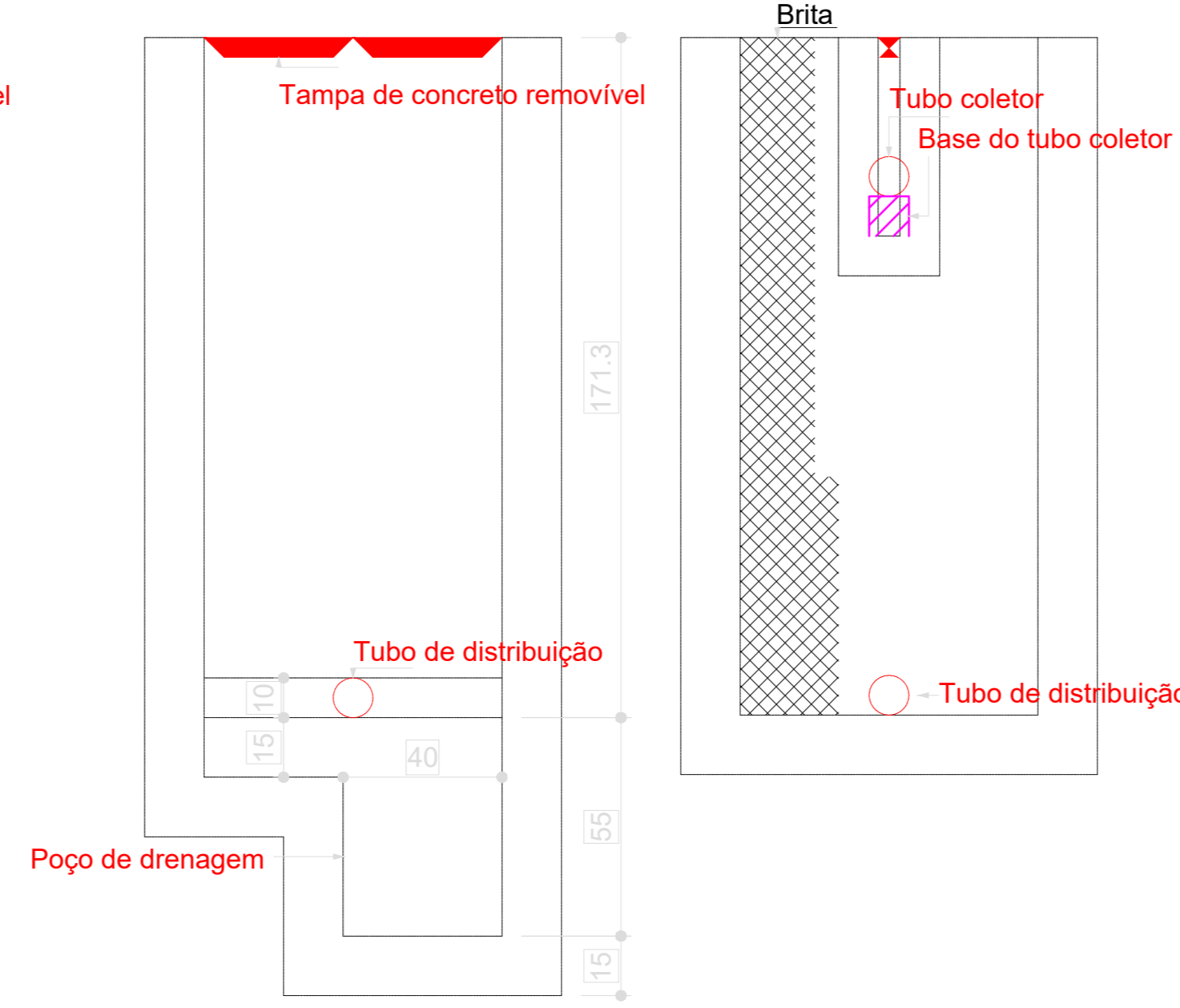
Filtro anaeróbio Corte 2 - ESC. 1:25
