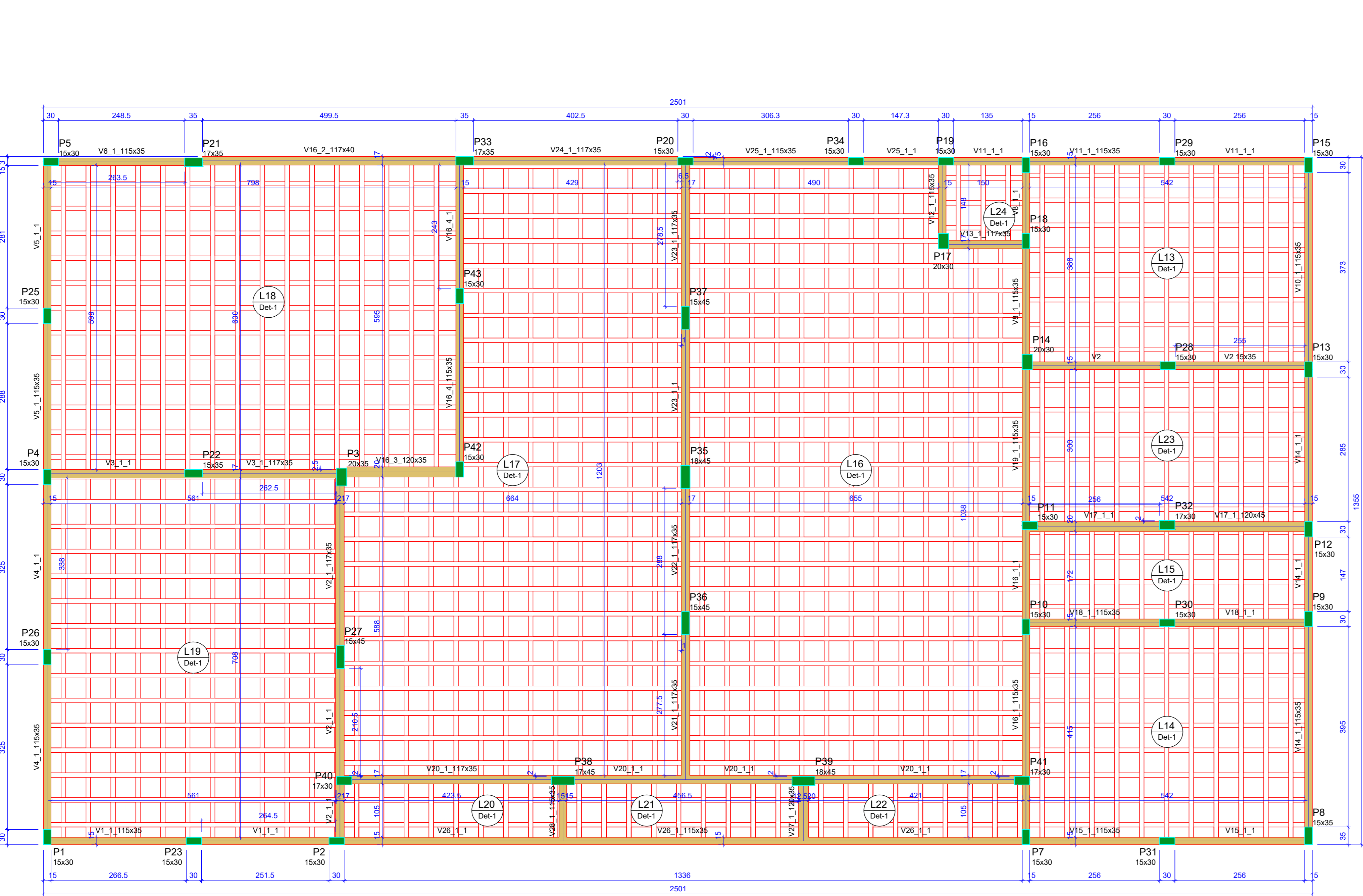
Forma do pavimento 1 PAVIMENTO escala 1:50
