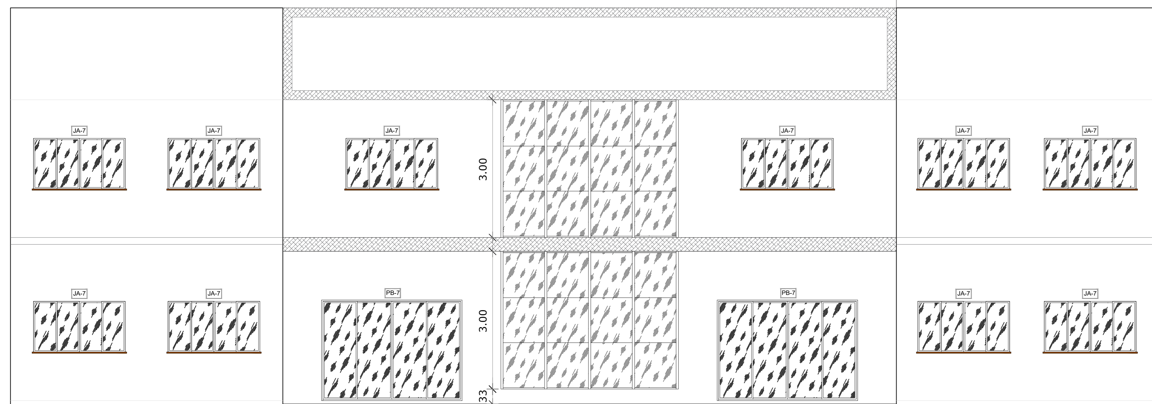
FACHADA 1 ESCALA 1/50
