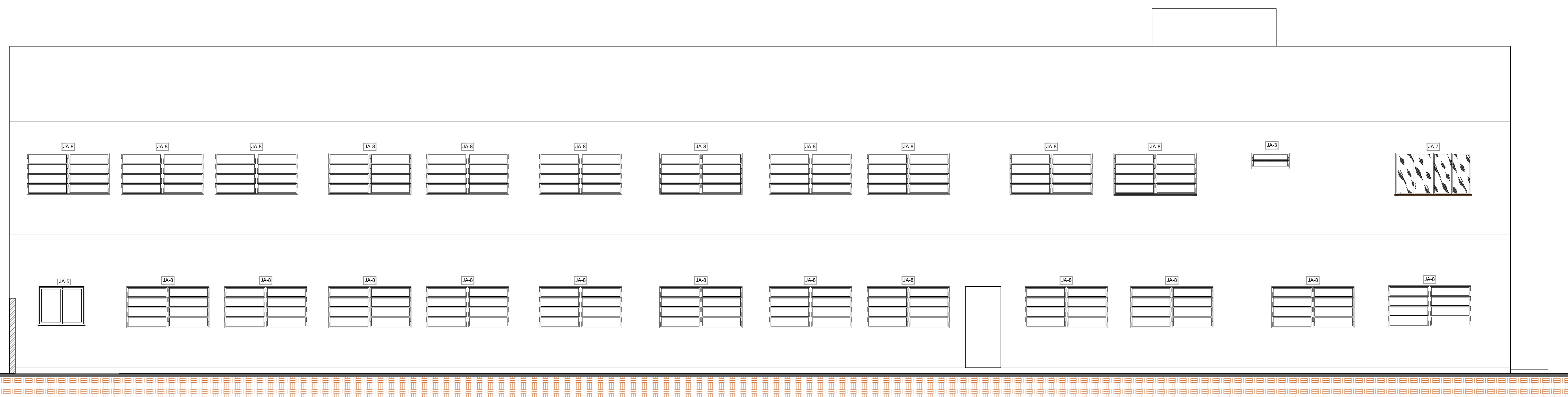
FACHADA 4 ESCALA 1/50
